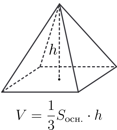
Объём пирамиды
