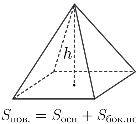
Площадь поверхности пирамиды
