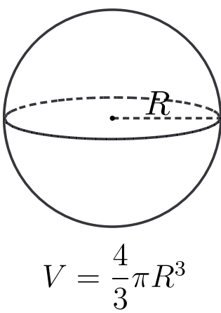
Объём шара
