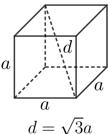
Диагональ прямоугольного параллелепипеда
