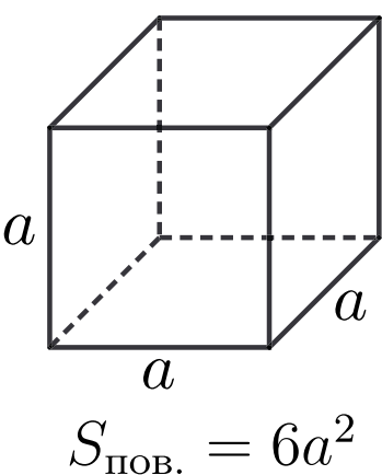
Площадь поверхности прямоугольного параллелепипеда
