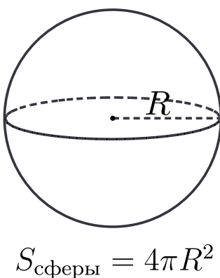
Площадь поверхности шара
