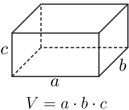
Объём прямой призмы
