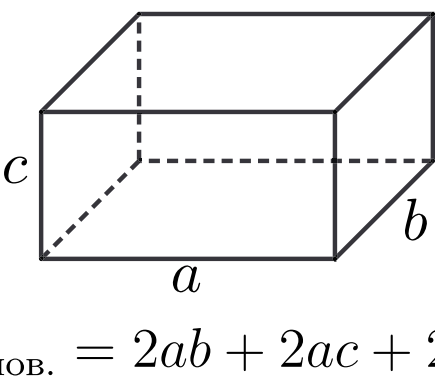
Площадь поверхности прямой призмы
