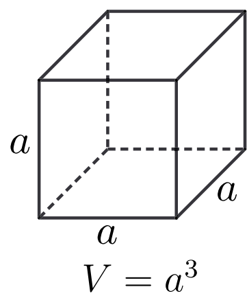
Объём прямоугольного параллелепипеда
